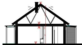
PRZEKRÓJ
