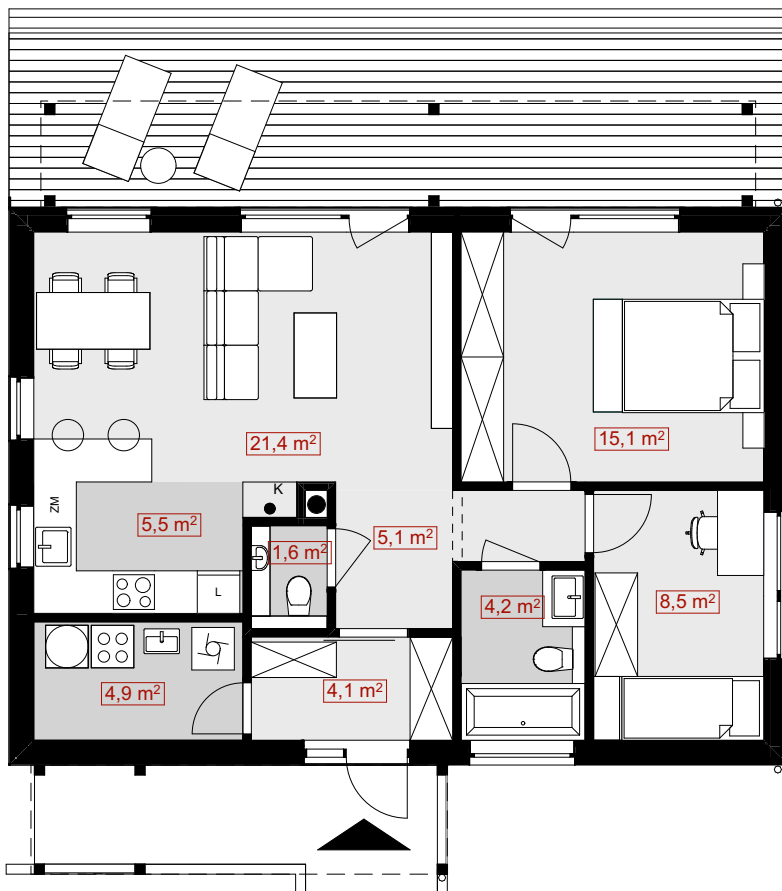
RZUT
